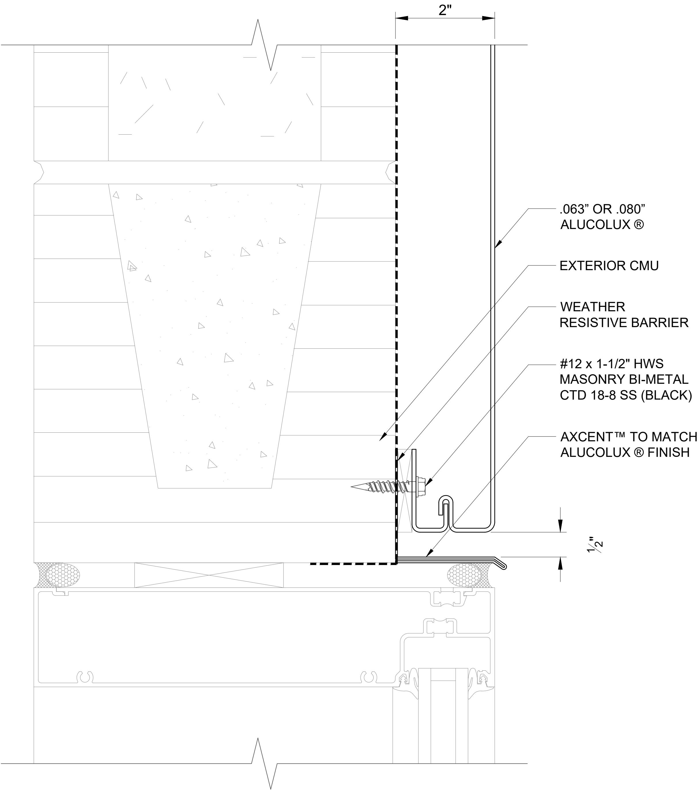
411 WINDOW HEAD SCALE: 3" = 1' - 0"
