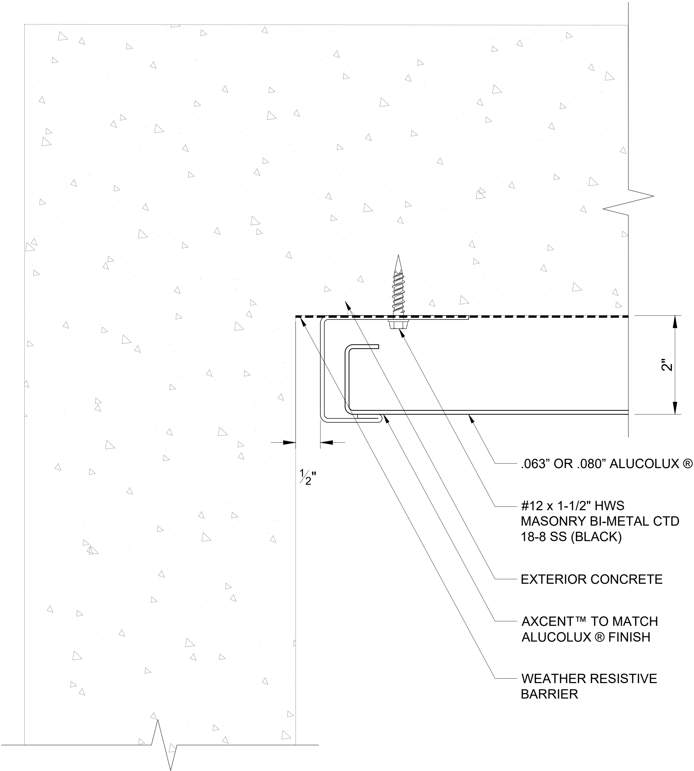
504 END WALL SCALE: 3" = 1' - 0"
