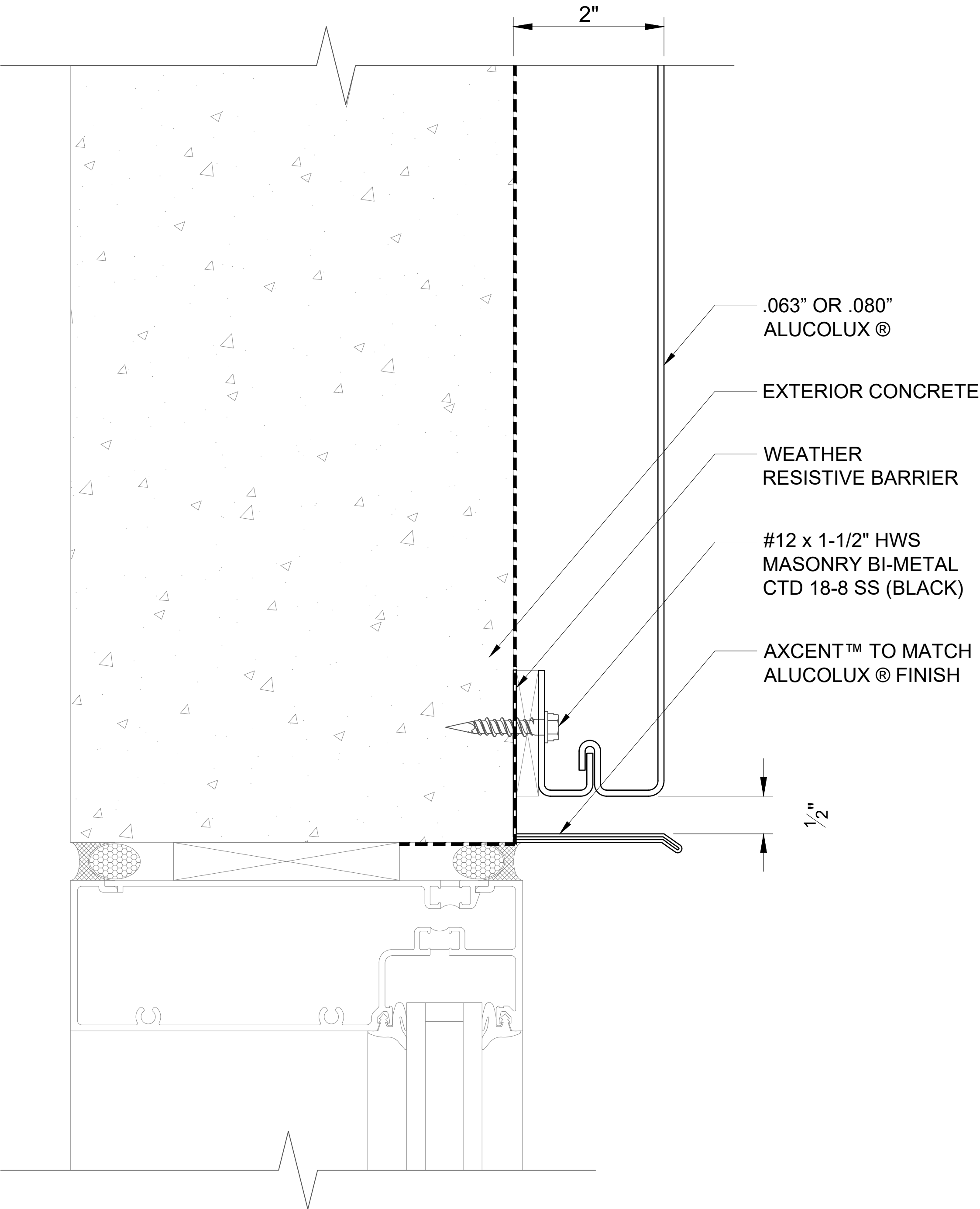
512 INSET WINDOW HEAD SCALE: 3" = 1' - 0"
