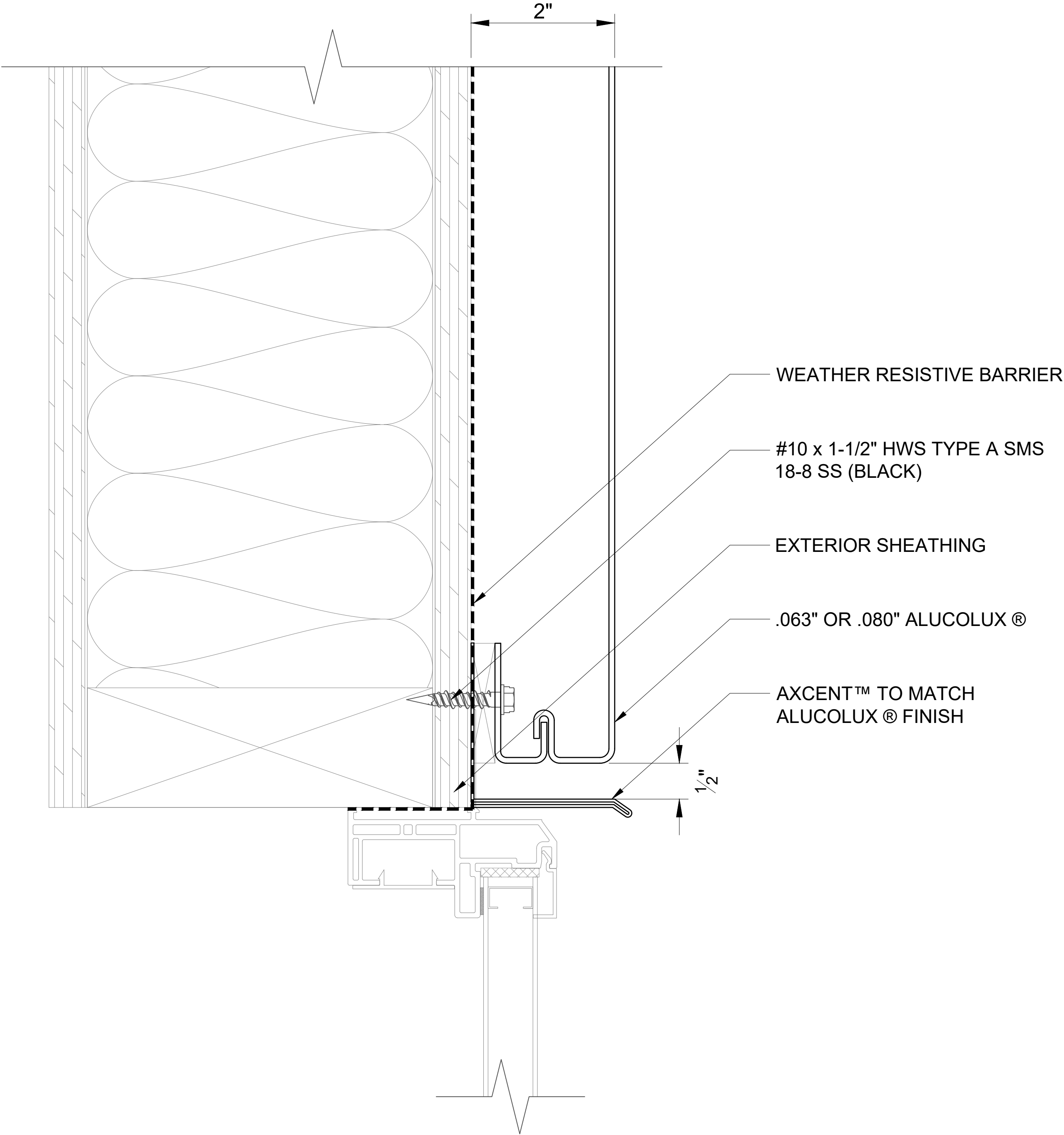
312 WINDOW HEAD SCALE: 3" = 1' - 0"
