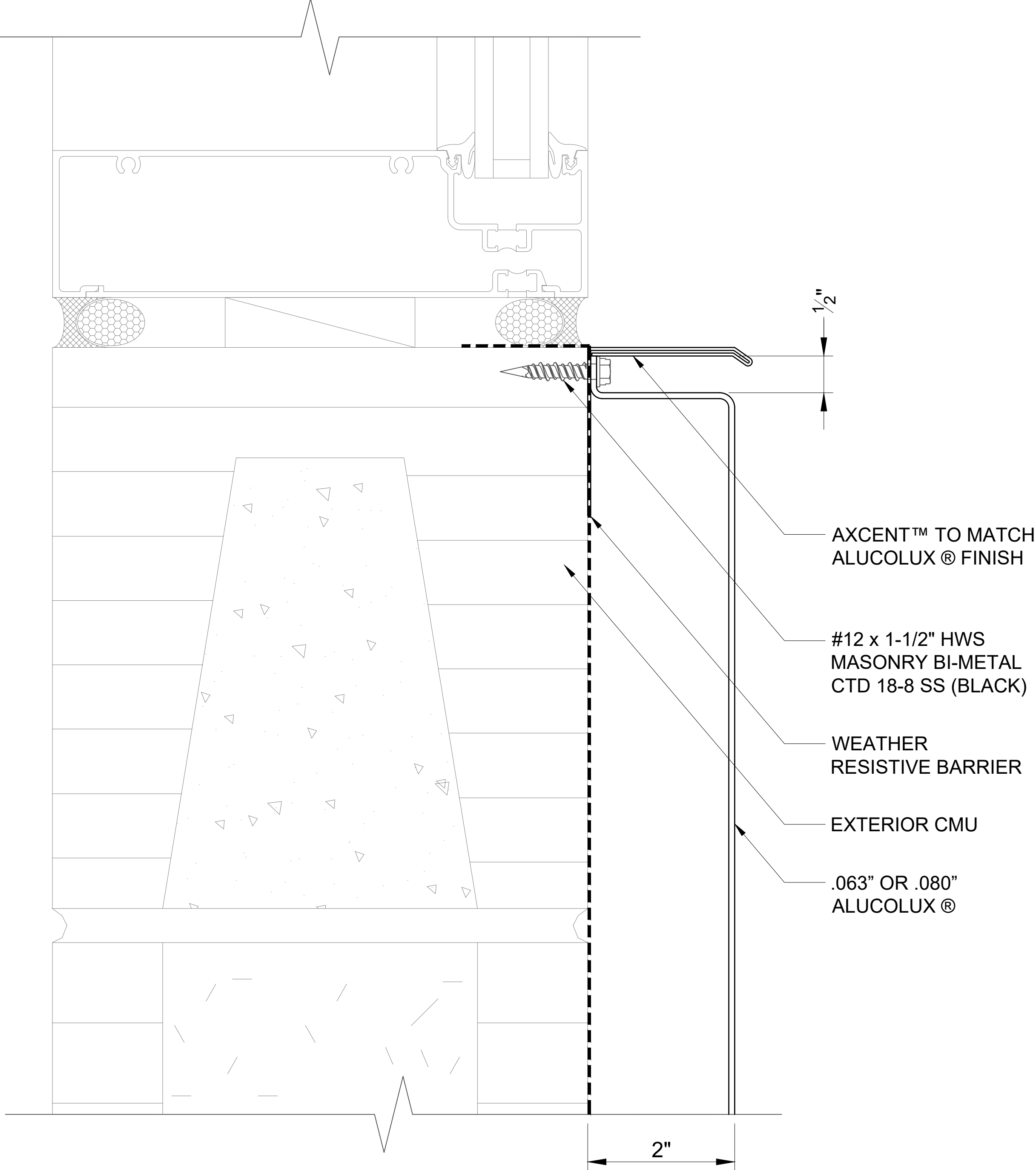
414 INSET WINDOW SILL SCALE: 3" = 1' - 0"
