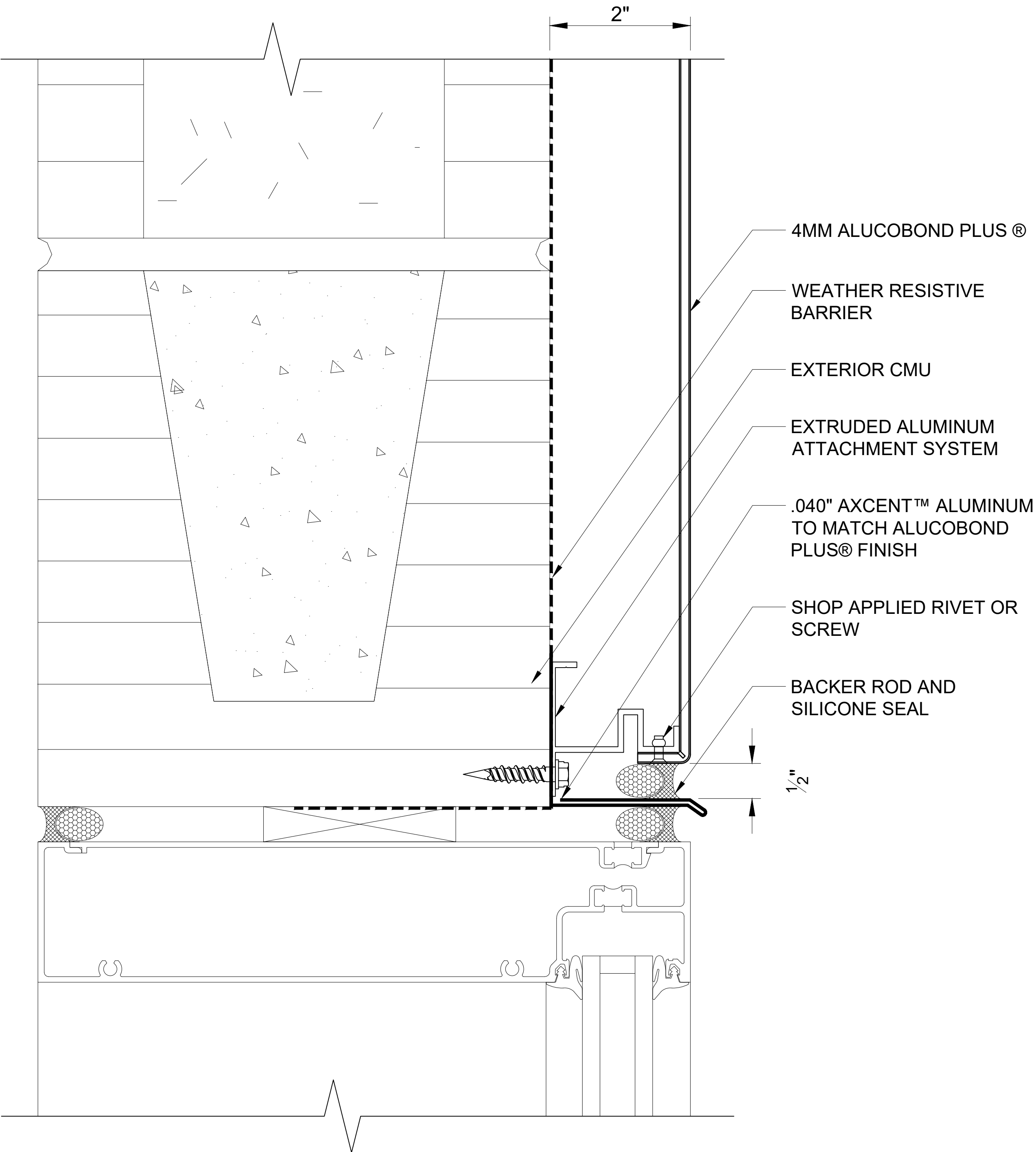
314 WINDOW HEAD SCALE: 3" = 1' - 0"
