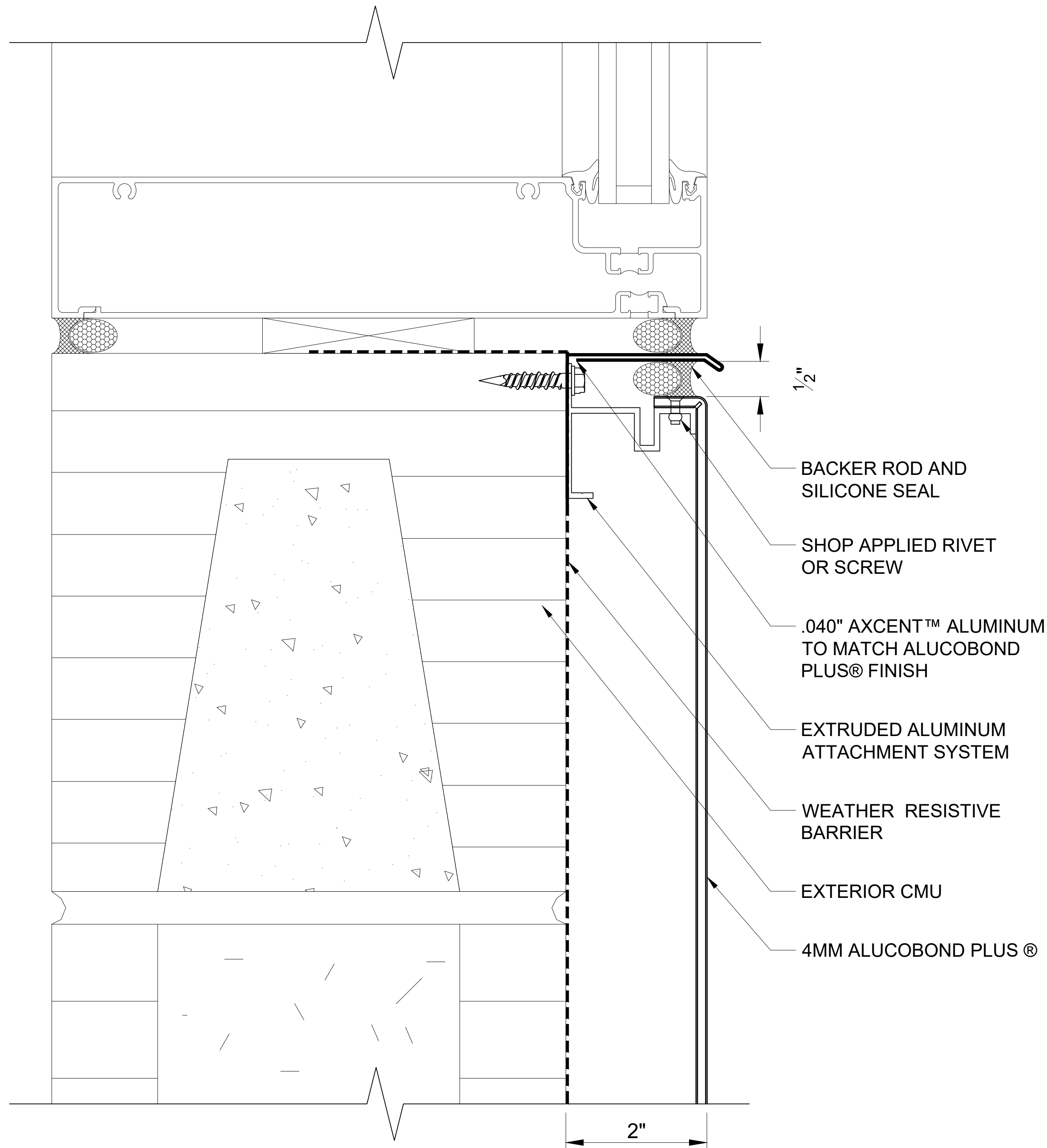
316 WINDOW SILL SCALE: 3" = 1' - 0"
