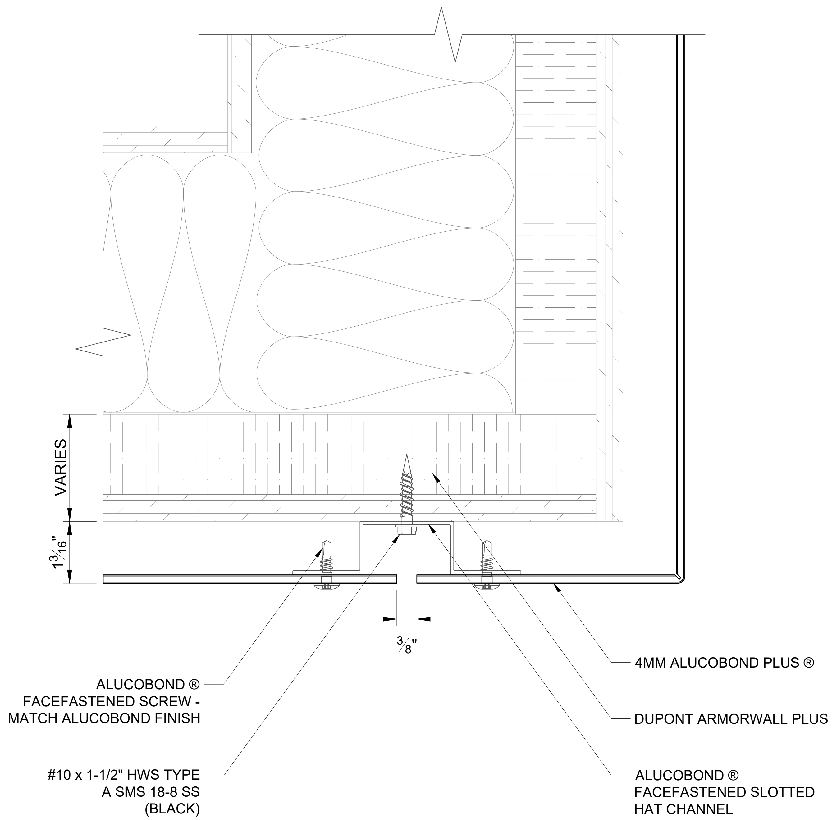
603 WALL TO SOFFIT SCALE: 3" = 1' - 0"
