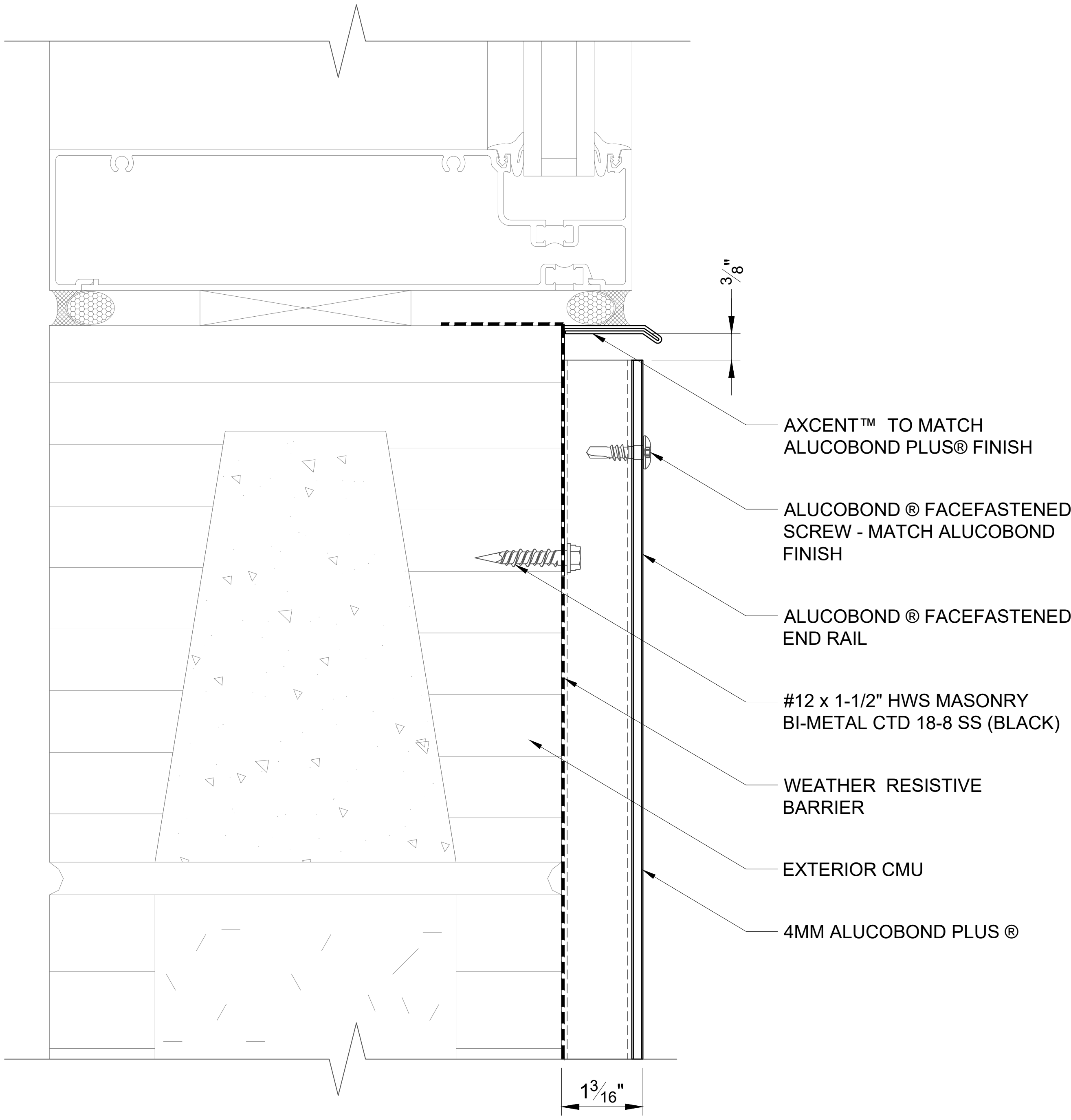
413 WINDOW SILL SCALE: 3" = 1' - 0"
