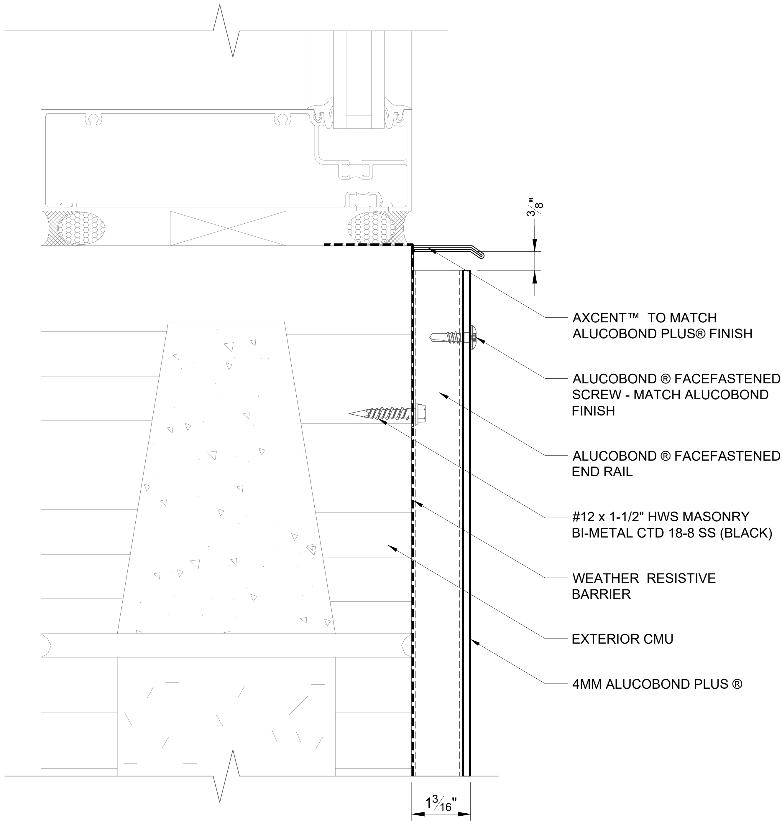
414 INSET WINDOW SILL SCALE: 3" = 1' - 0"
