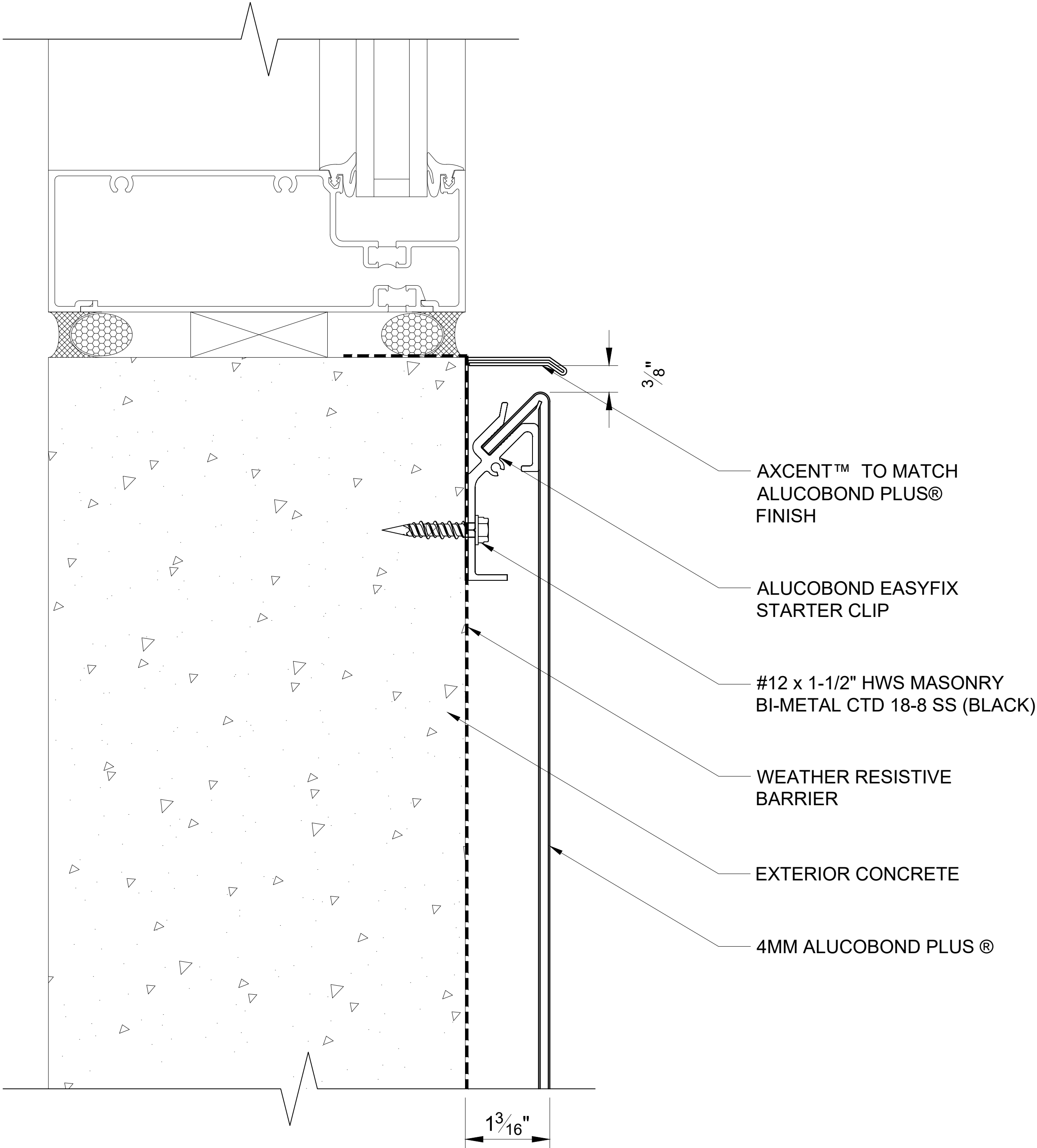
513 INSET WINDOW SILL SCALE: 3" = 1' - 0"
