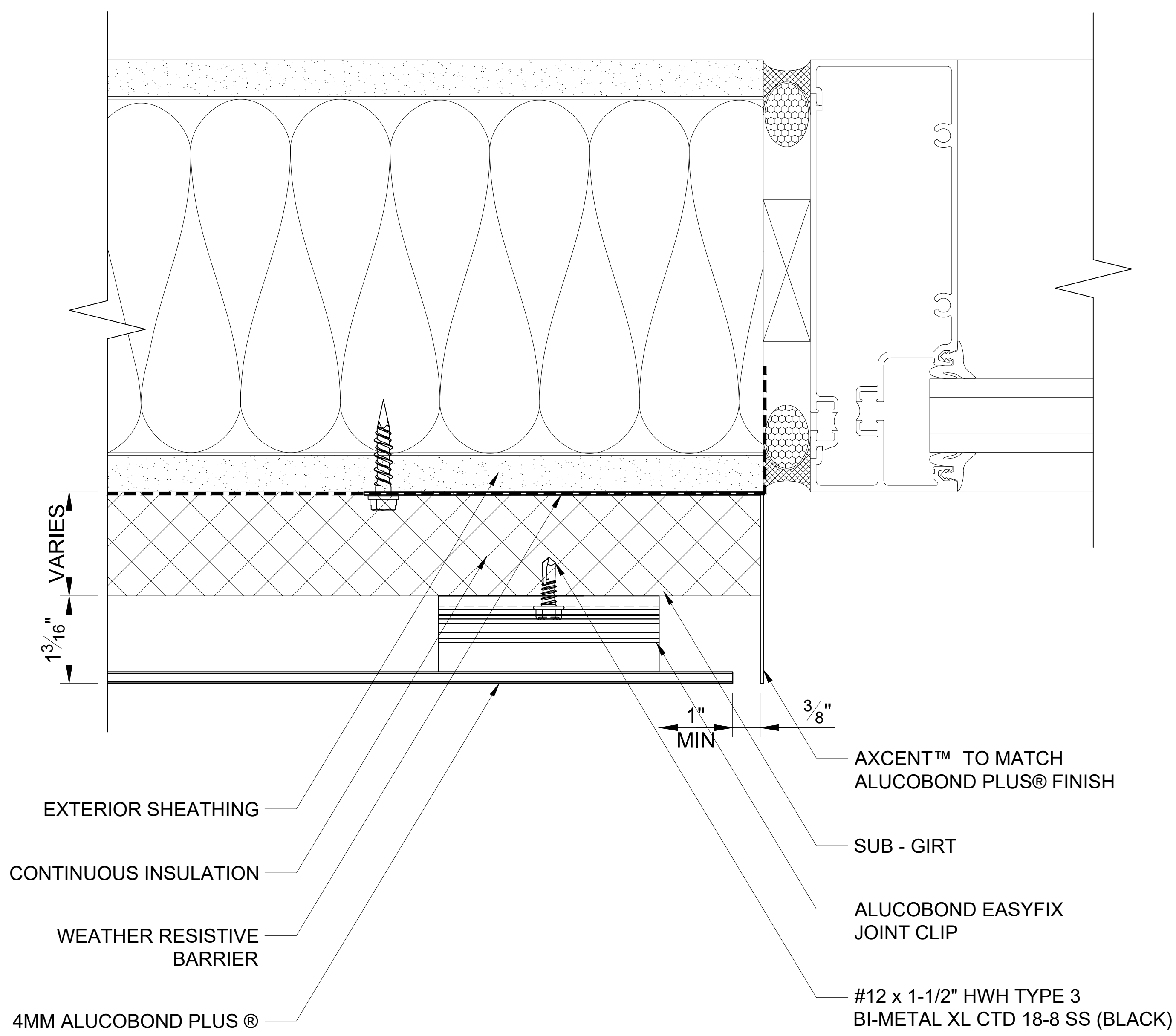
115 INSET WINDOW JAMB SCALE: 3" = 1' - 0"
