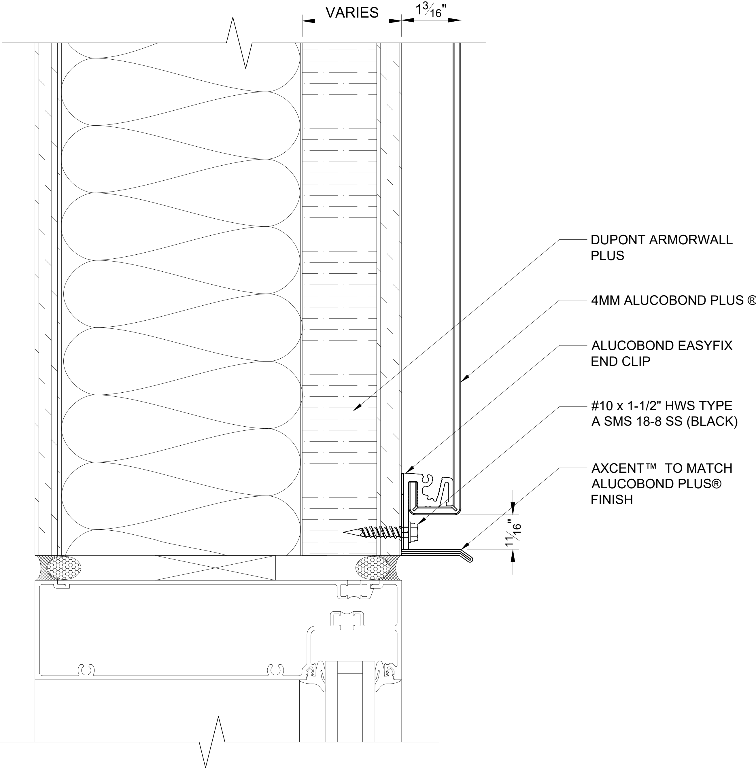
611 INSET WINDOW HEAD SCALE: 3" = 1' - 0"
