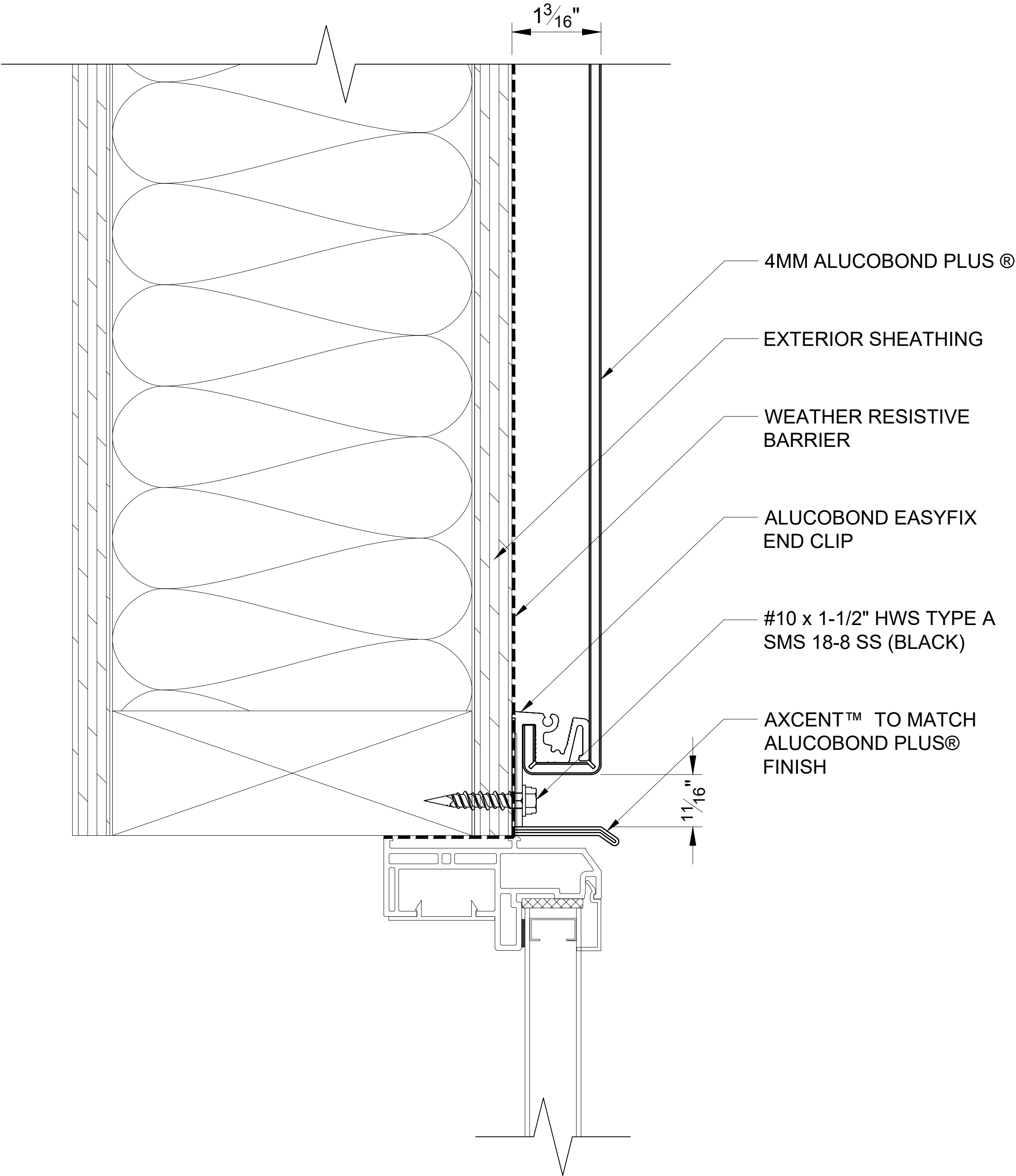
311 WINDOW HEAD SCALE: 3" = 1' - 0"
