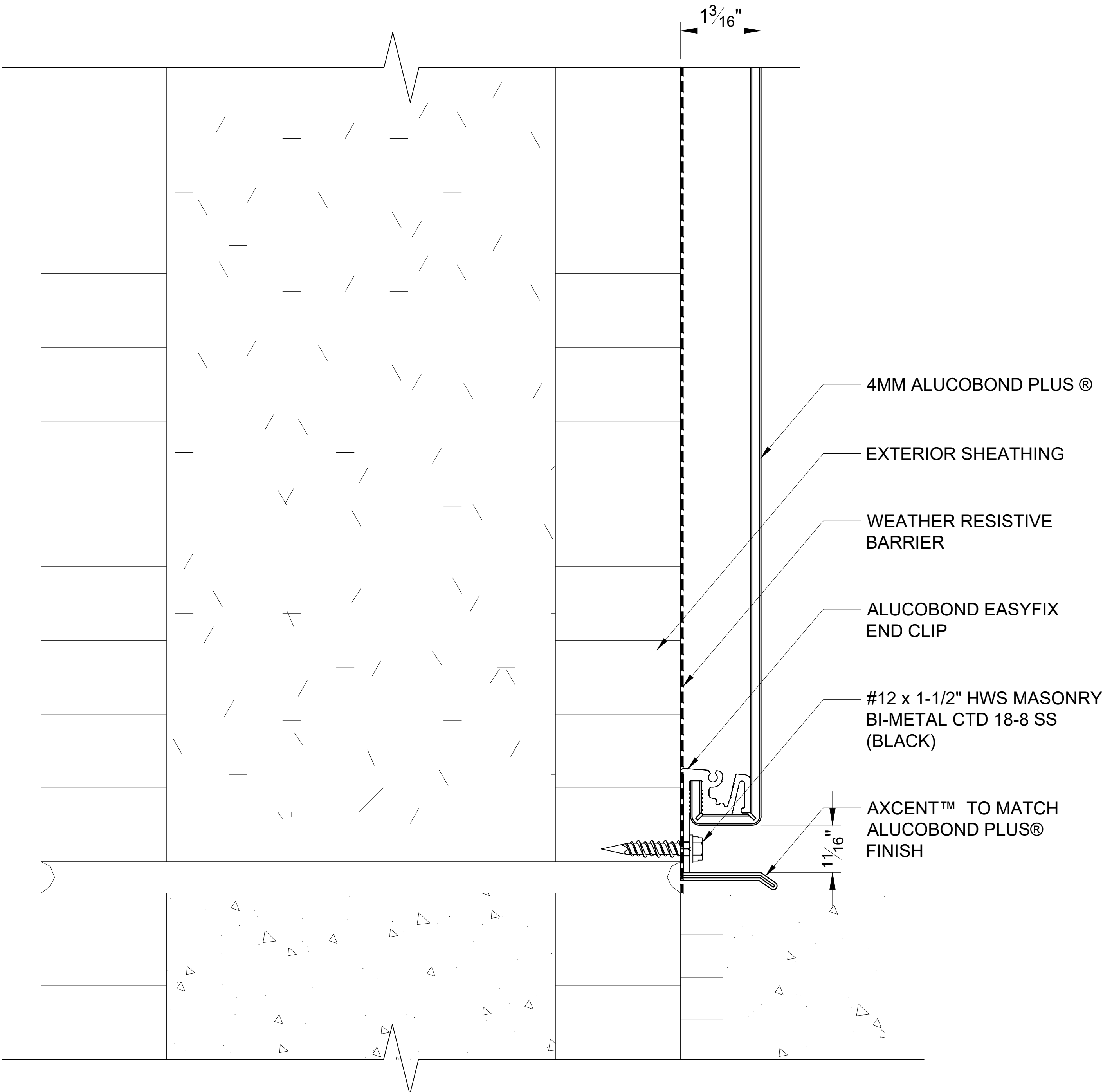
406 BASE SCALE: 3" = 1' - 0"
