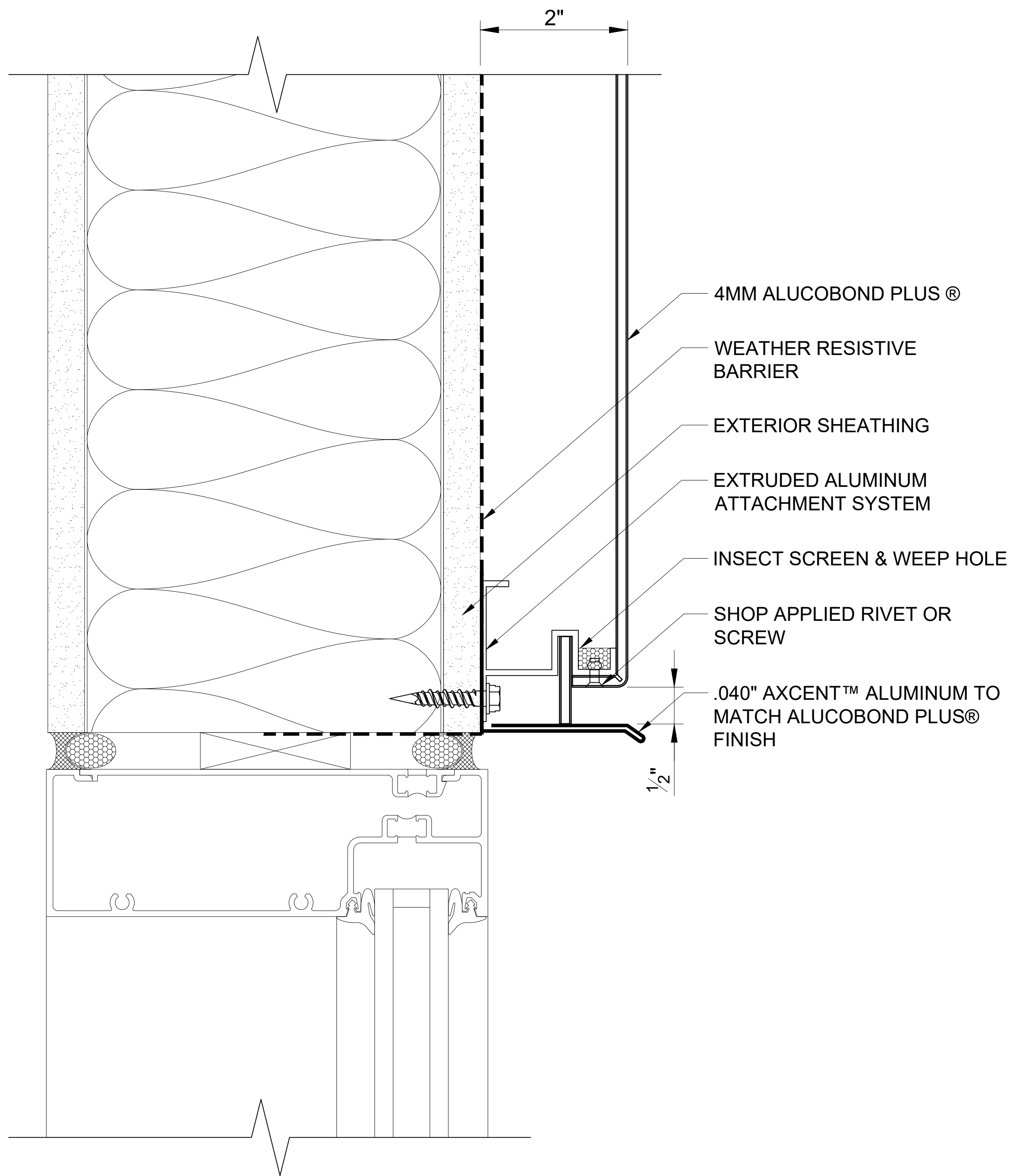
215 INSET WINDOW HEAD SCALE: 3" = 1' - 0"
