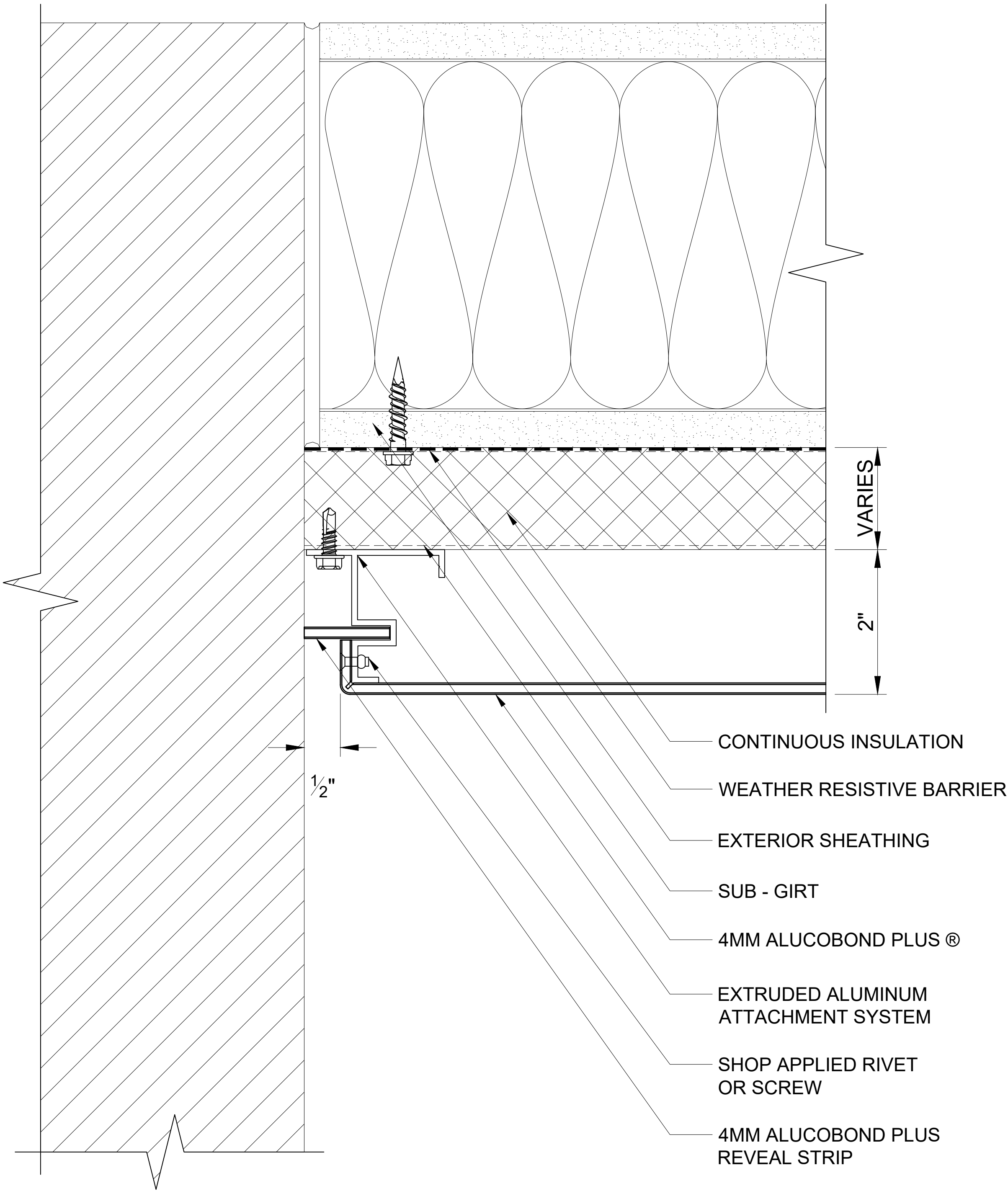
107 END WALL - PLAN VIEW SCALE: 3" = 1' - 0"
