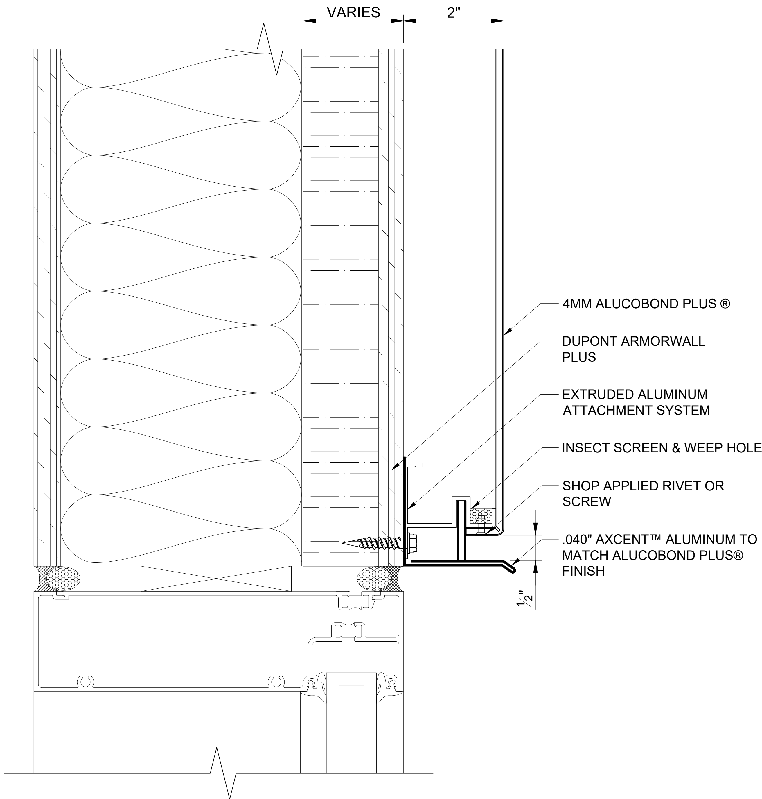
515 INSET WINDOW HEAD SCALE: 3" = 1' - 0"
