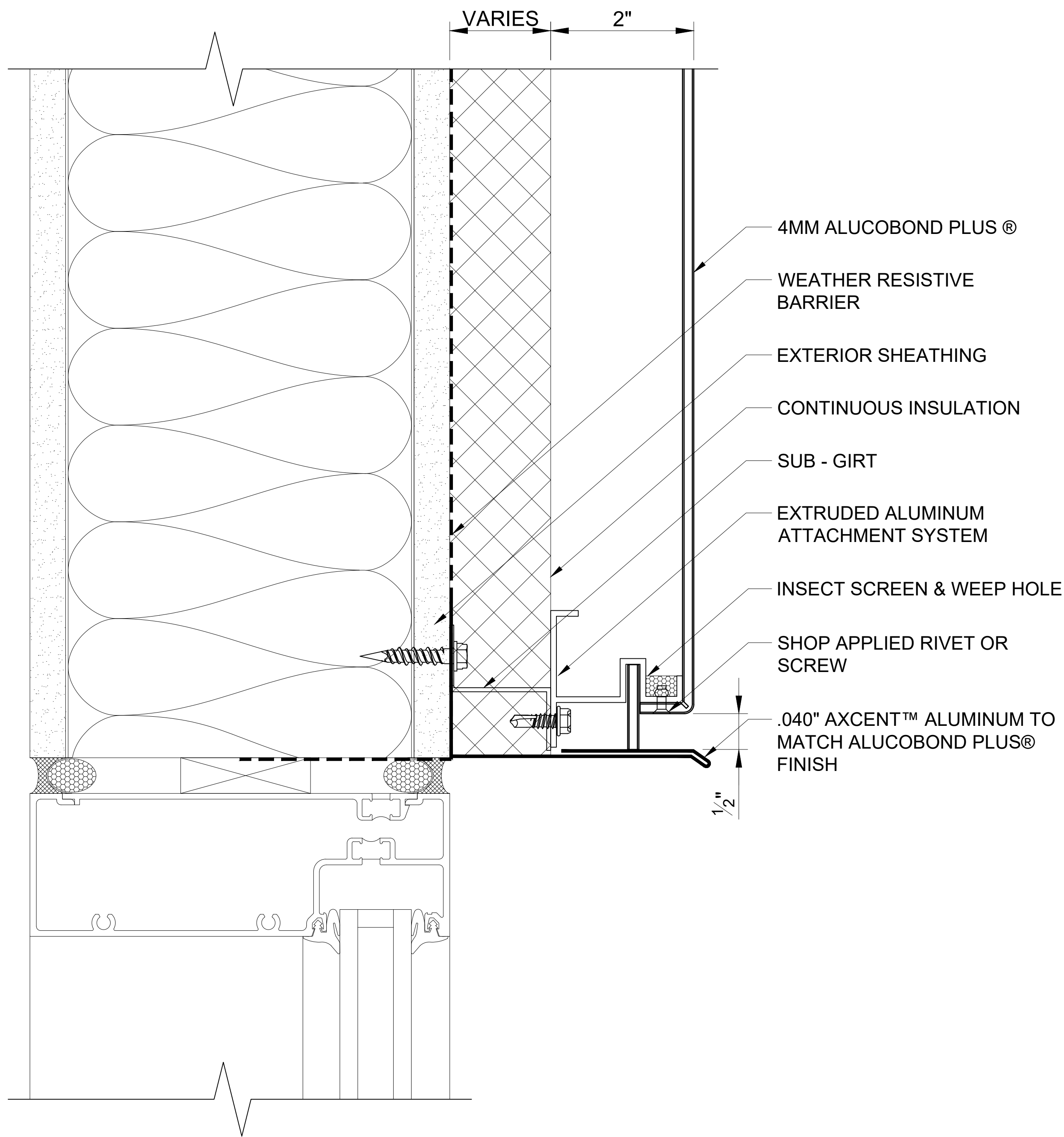
115 INSET WINDOW HEAD SCALE: 3" = 1' - 0"
