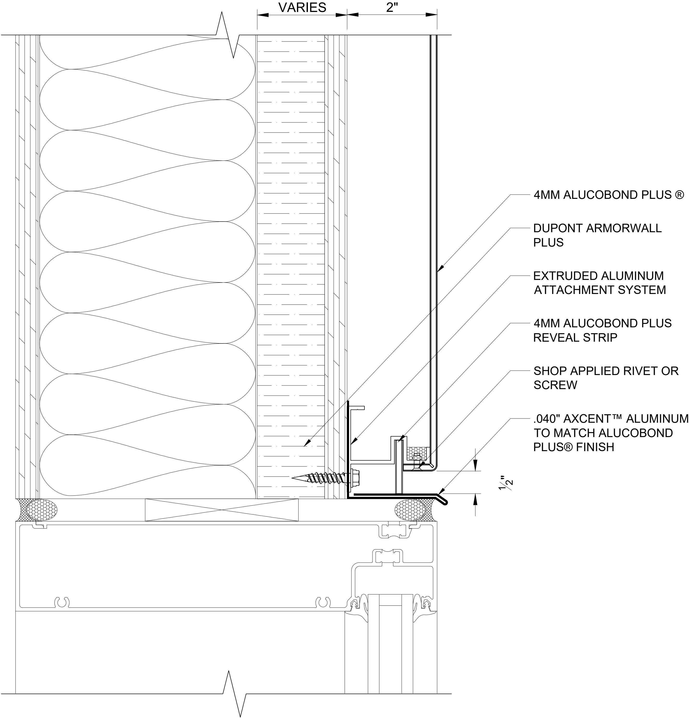
514 WINDOW HEAD SCALE: 3" = 1' - 0"
